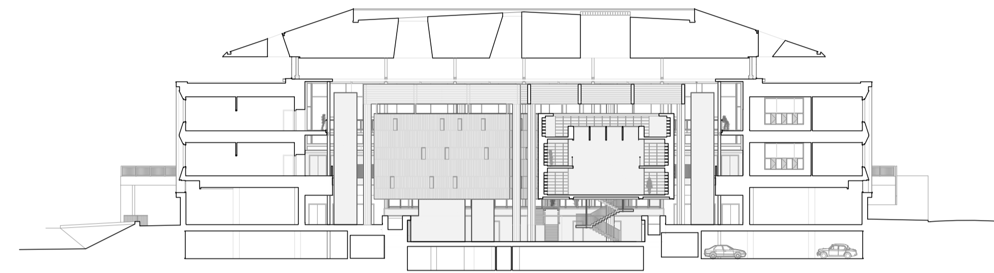
SECCIÓN B-B'
