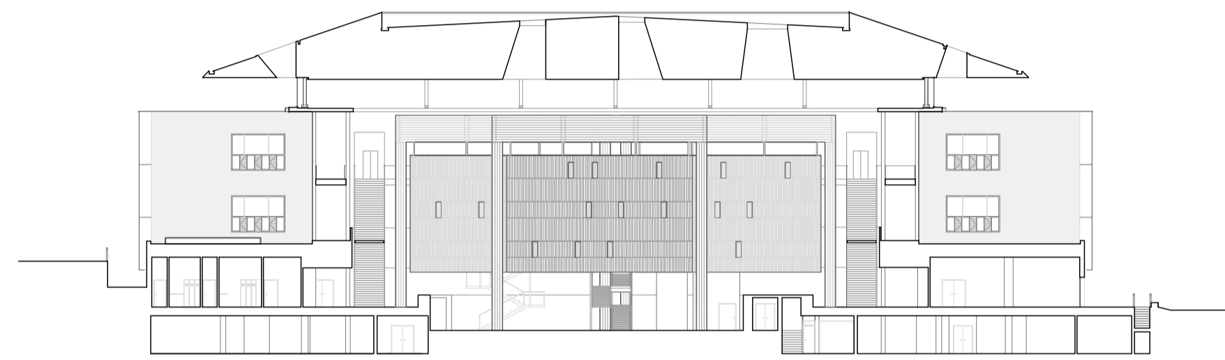
SECCIÓN A-A'
