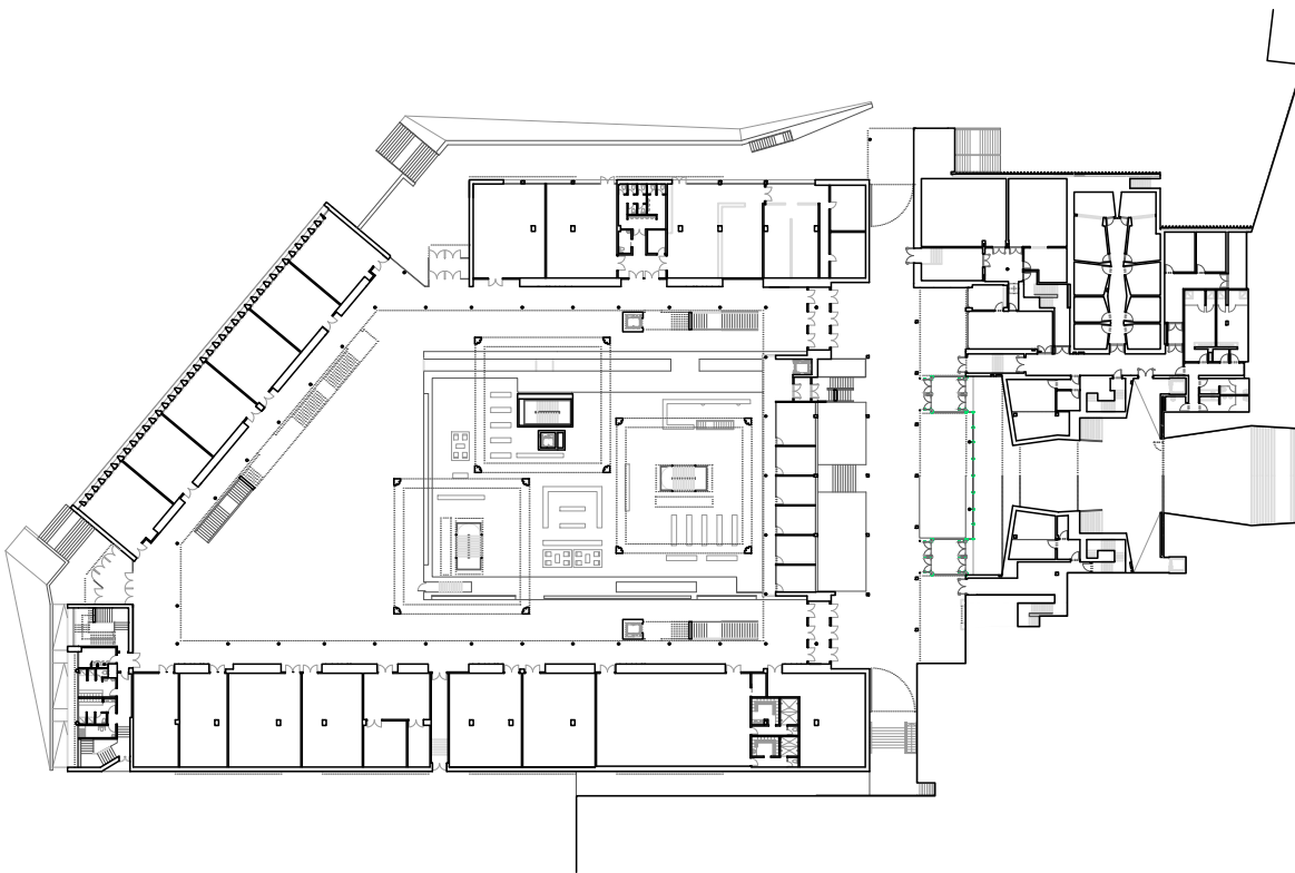
PLANTA BAJA
