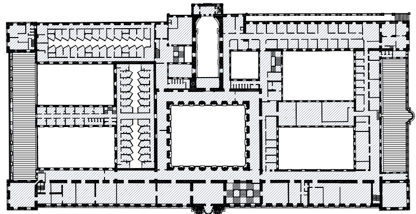
PLANTA ALTA ESTADO PREVIO 1990 ANTERIOR A LA PRIMERA FASE
