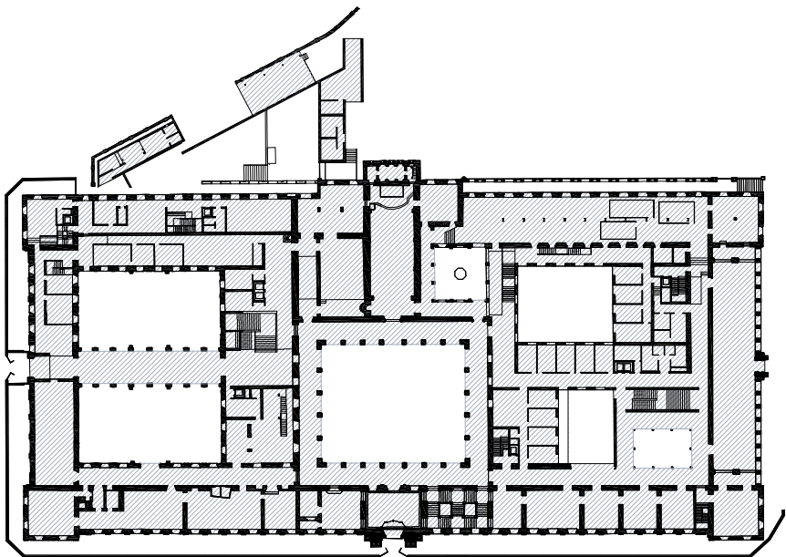
PLANTA BAJA PROPUESTA. 2005
