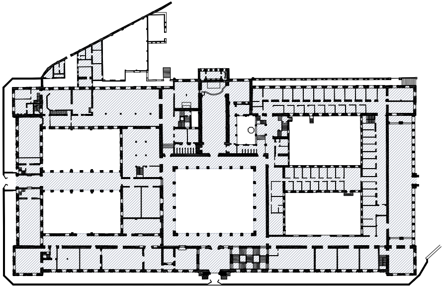
PLANTA BAJA ESTADO PREVIO 1990 ANTERIOR A LA PRIMERA FASE
