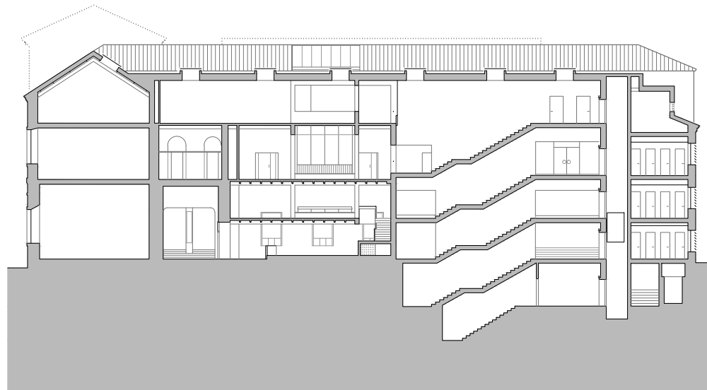
SECCIÓN TRANSVERSAL POR ESCALERA PRINCIPAL
