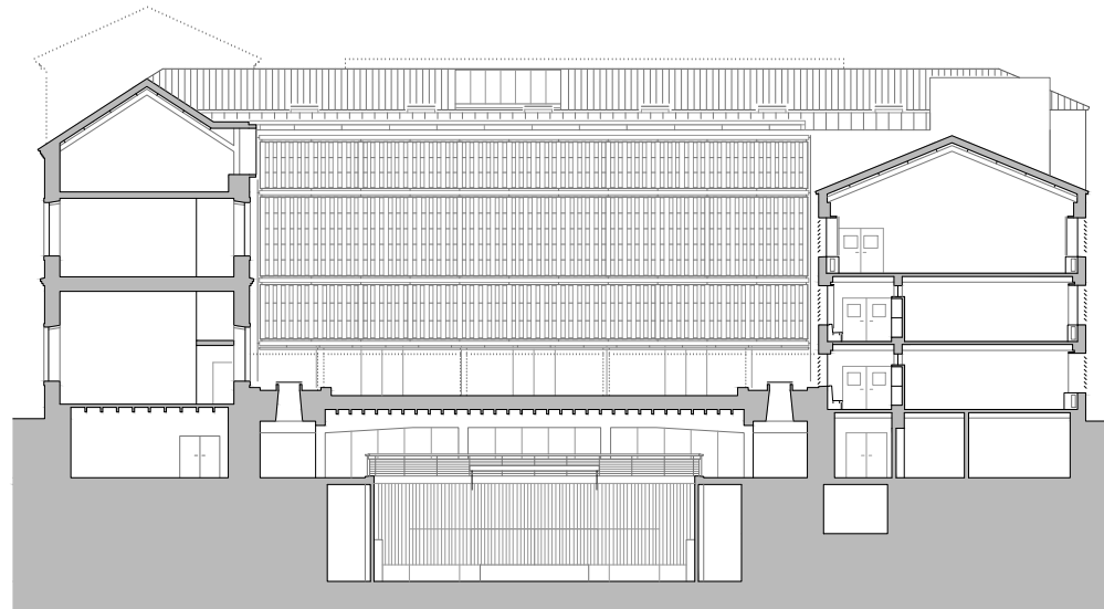
SECCIÓN TRANSVERSAL POR AULA MAGNA
