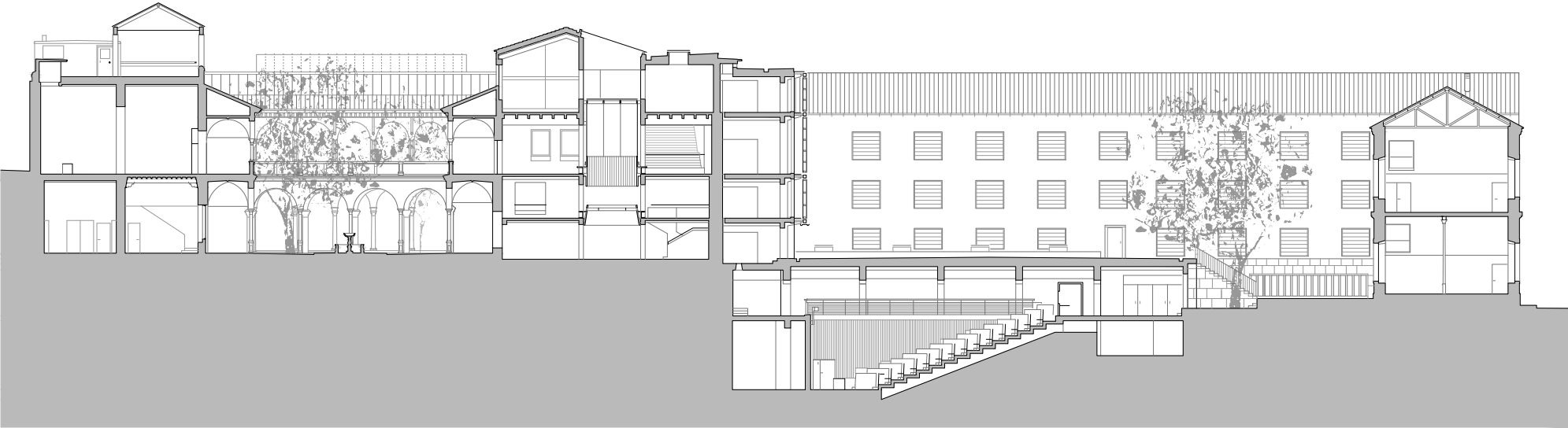
SECCIÓN LONGITUDINAL POR AULA MAGNA
