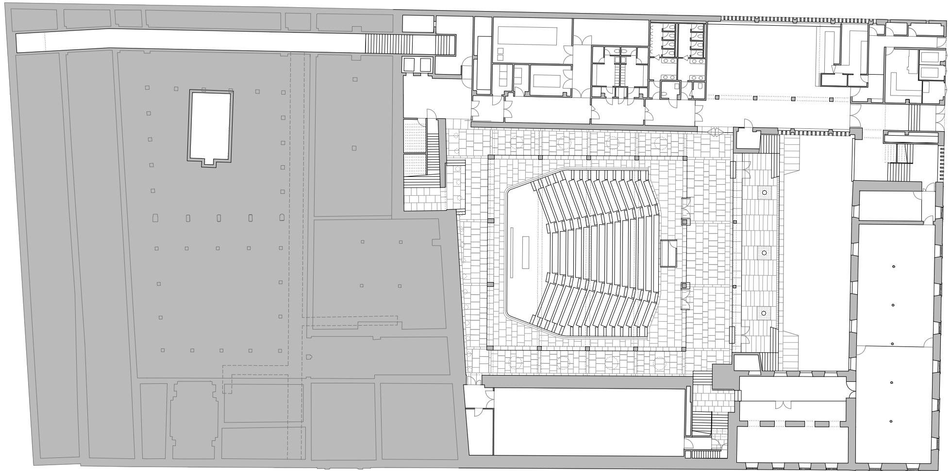
PLANTA SEMISÓTANO
