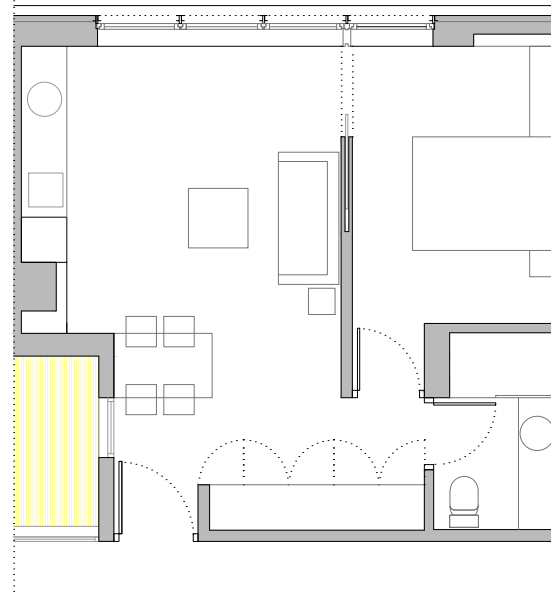
Apartamento de jóvenes 40 m 2 e: 1/100
