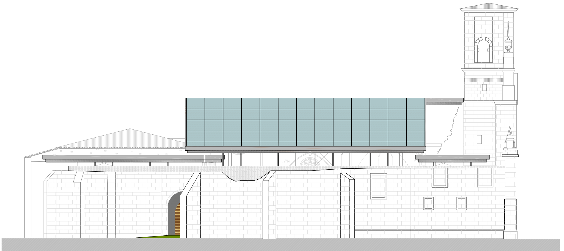
Alzado C
