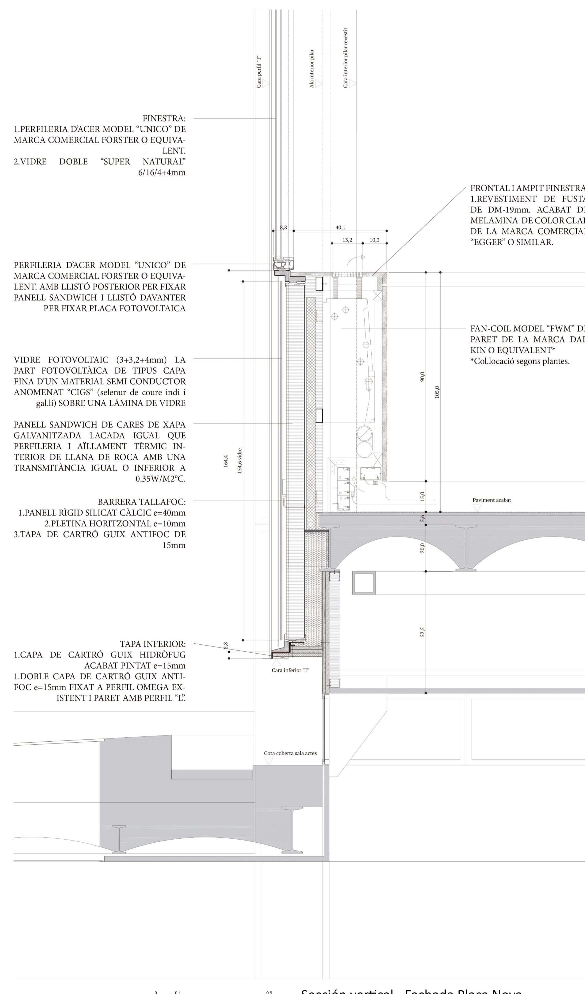
0 0.1 0.5 Sección vertical - Fachada Plaça Nova
