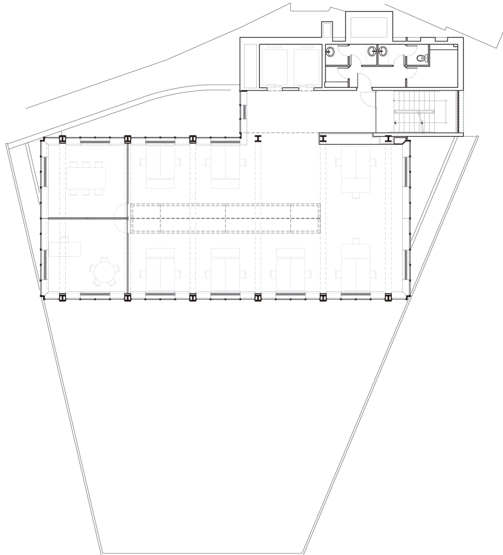
Planta segunda
