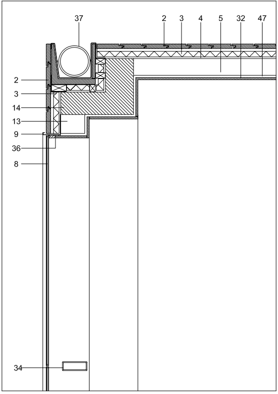
SECCION HORIZONTAL POR CANALON
