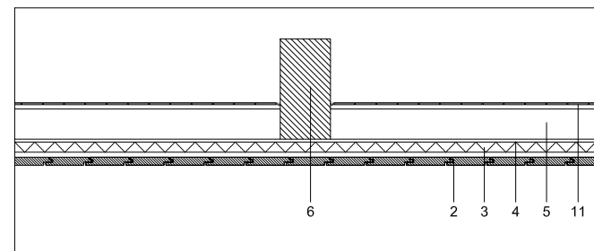
SECCION HORIZONTAL POR PILAR EN EL ESPACIO DE LA PISCINA
