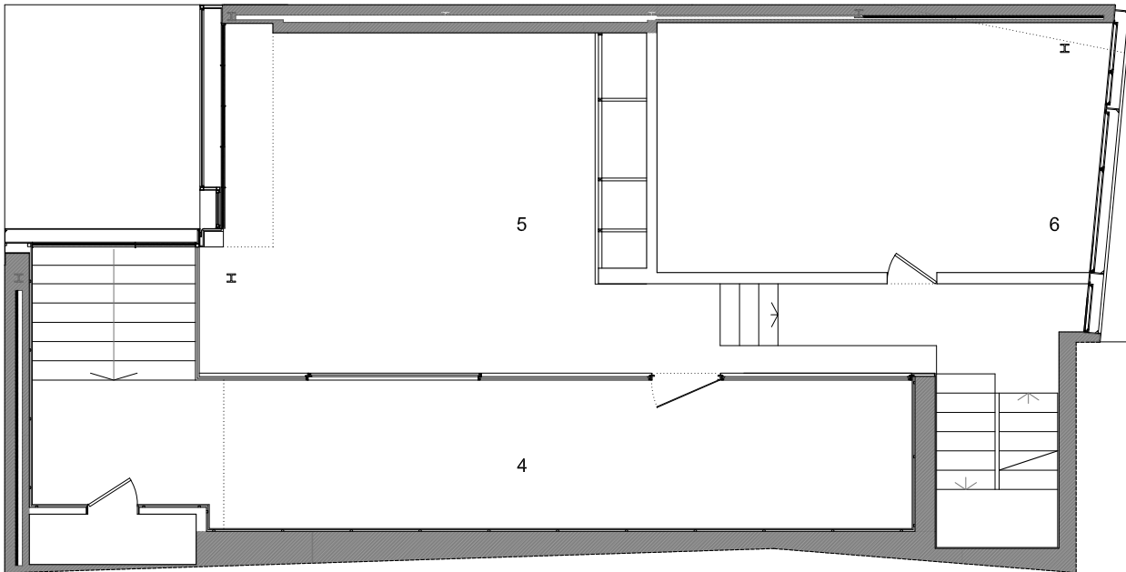
planta baja
