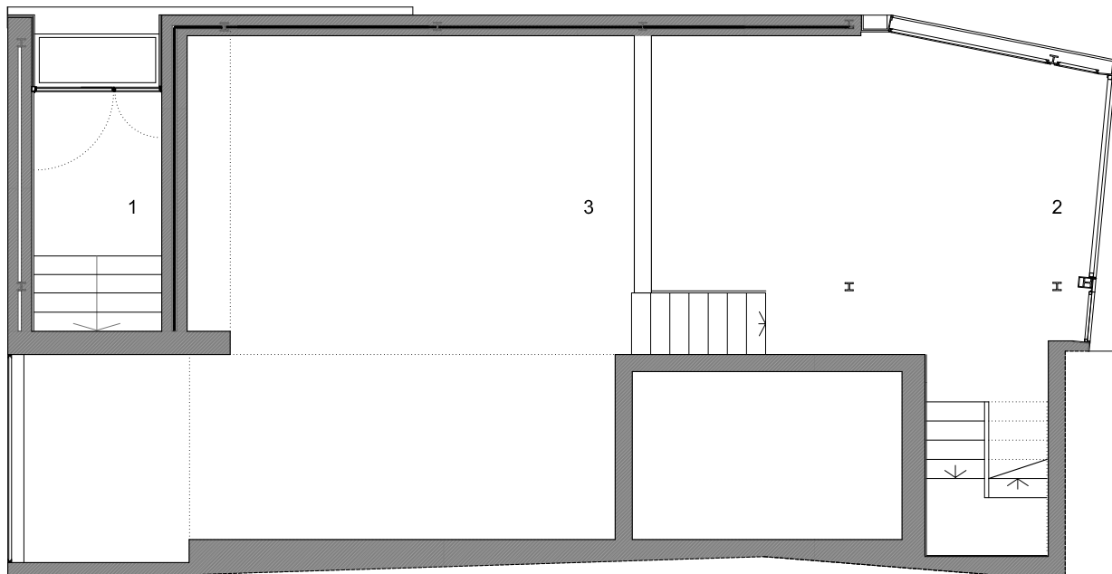
planta sotano
