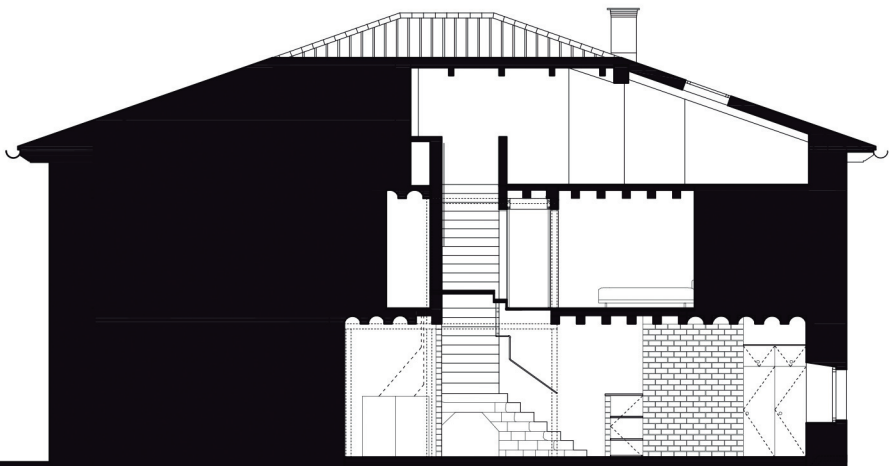
SECCIÓN CC¹
