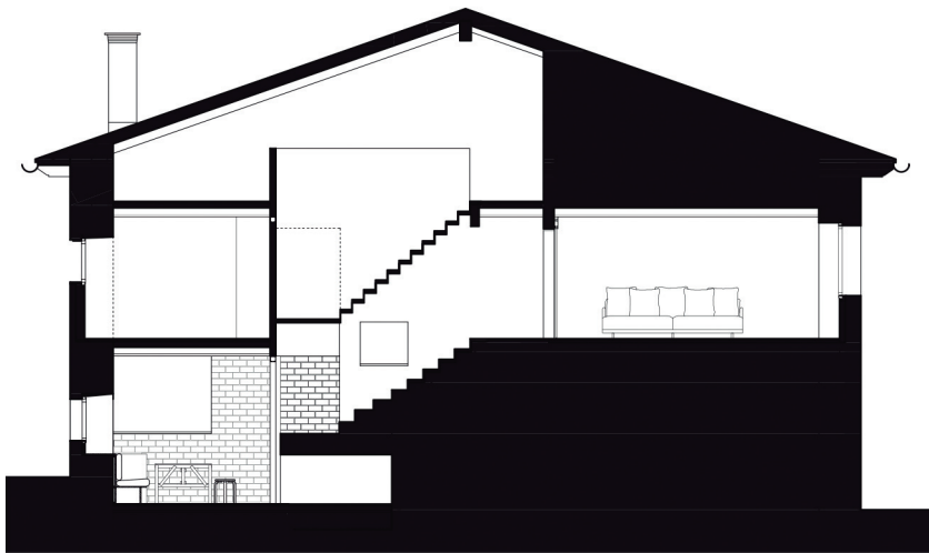
SECCIÓN BB'
