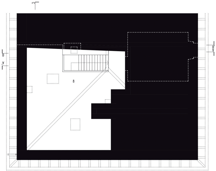
PLANTA BAJOCUBIERTA
