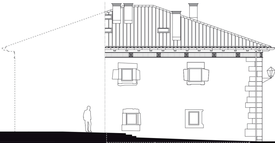
ALZADO NORTE
