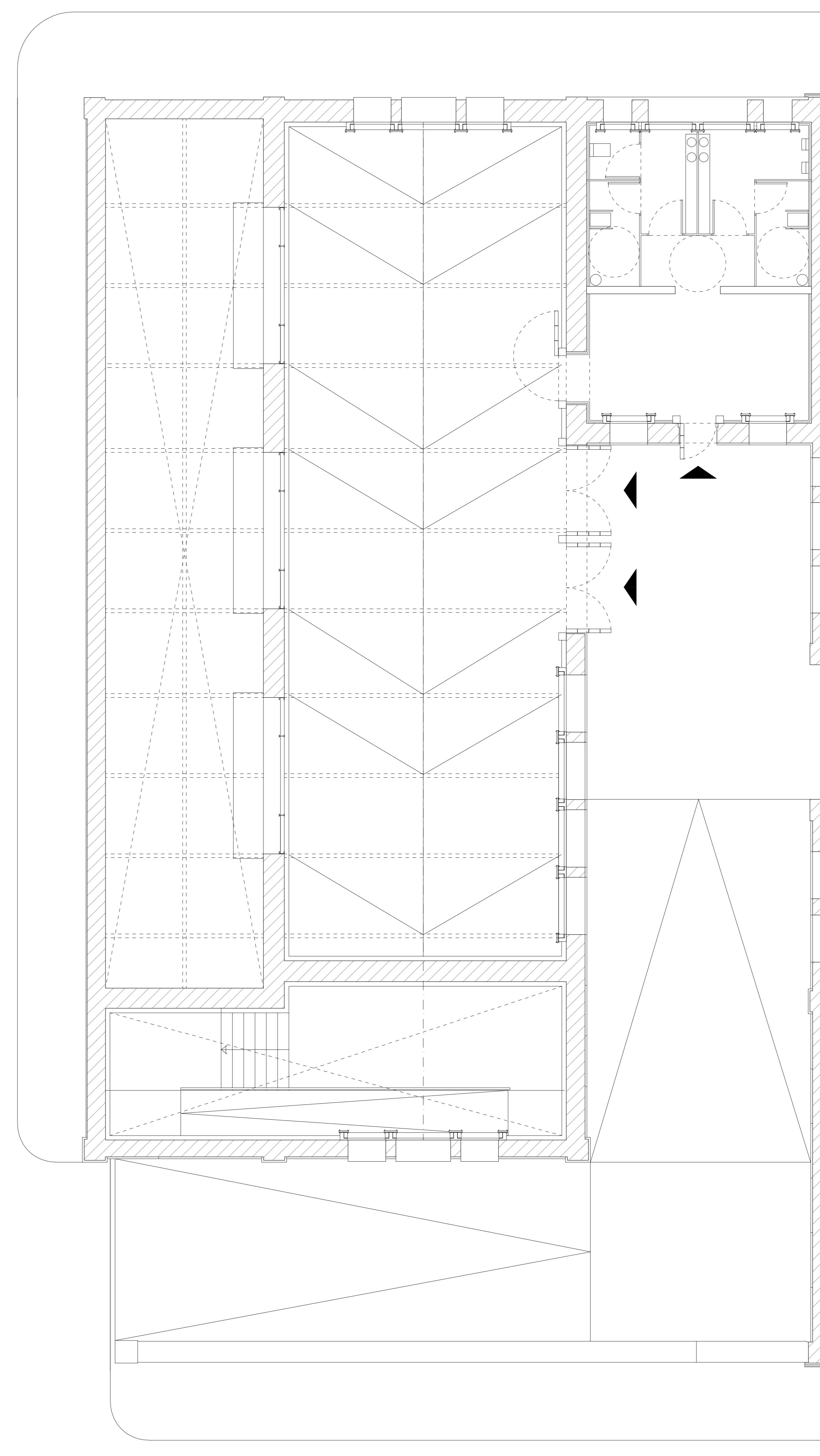
Planta primera
