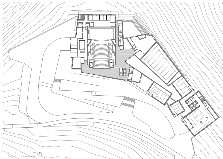
0 5 10 20 PLANTA PRIMERA / FIRST FLOOR PLAN
