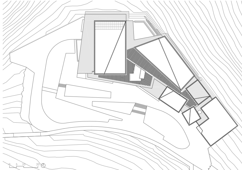
0 5 10 20 PLANTA CUBIERTAS / ROOF PLAN
