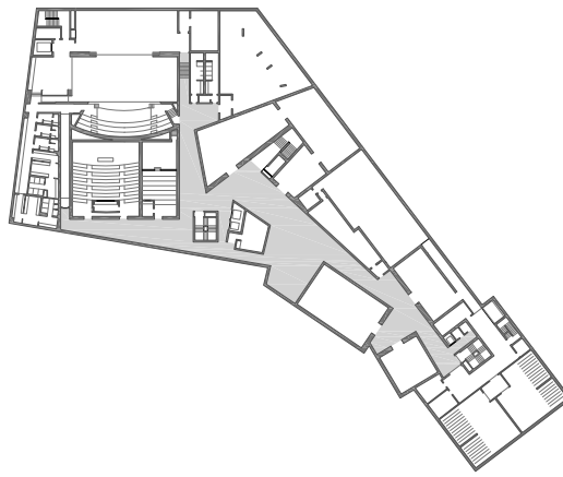
0 5 10 20 SÓTANO PRIMERO / FIRST BASEMENT
