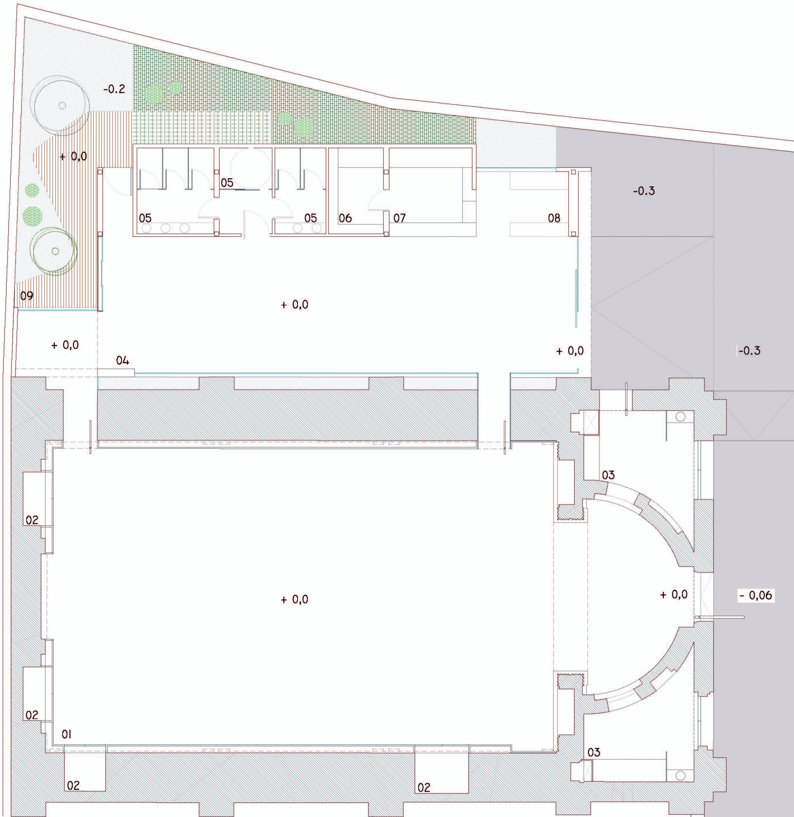
PLANTA NIVEL +I
