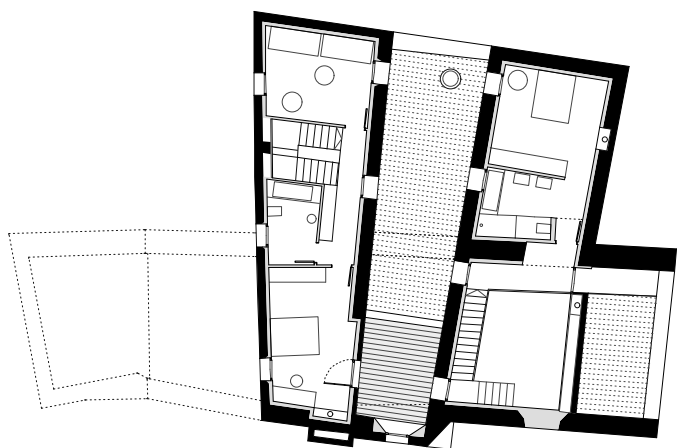
PLANTA NIVEL 1
