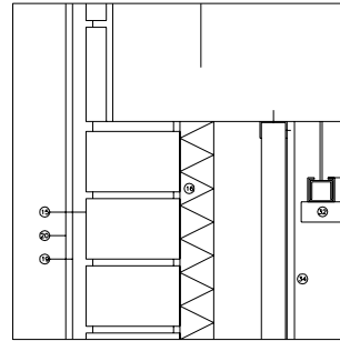
D3. ENTREGA FALS SOSTRE AMB TANCAMENT
