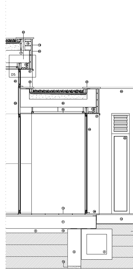
D5. REMAT SUPERIOR FUSTERIA BATENT
