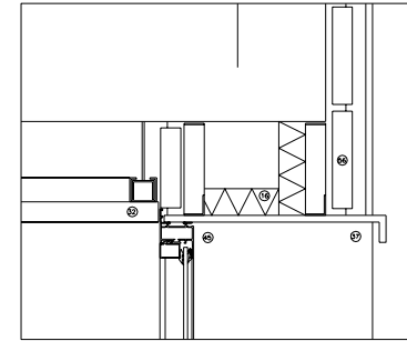
D5. REMAT SUPERIOR FUSTERIA BATENT
