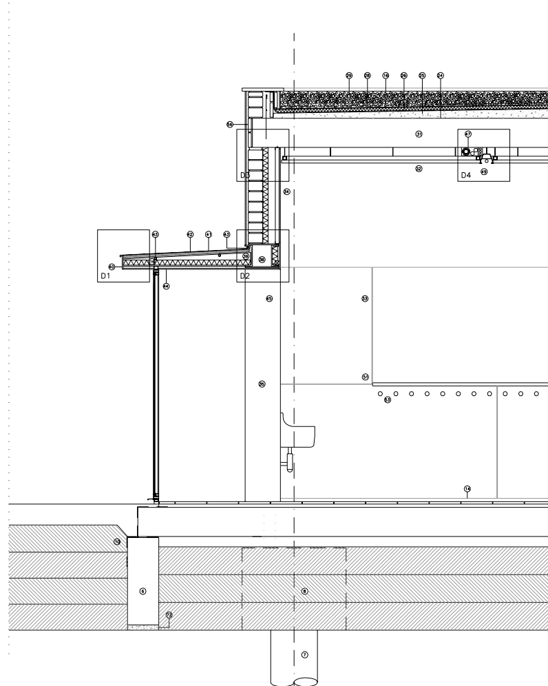
SECCIÓ AULA
