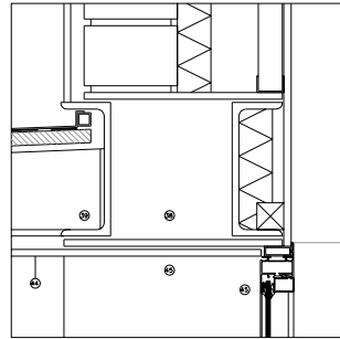
D2. ENTREGA RAFEC AMB TANCAMENT I FUSTERIA
