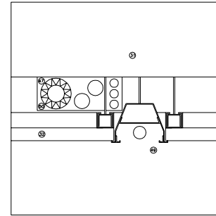
D4. ENTREGA FALS SOSTRE AMB LLUMENERA
