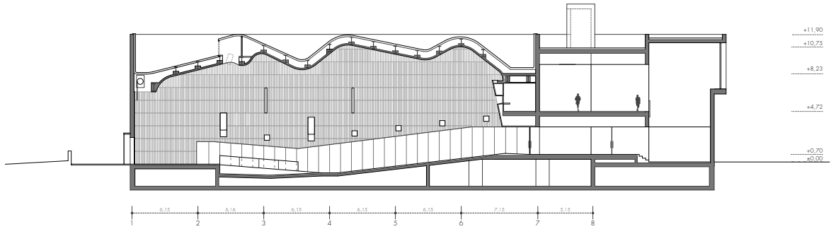
SECCIÓN 1. LONGITUDINAL POR SALA 1 LONGITUDINAL SECTION. MAIN HALL
