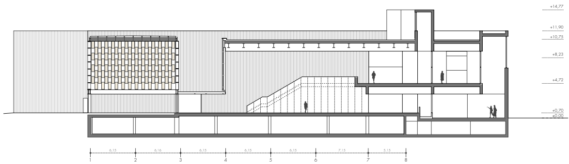
SECCIÓN 2. LONGITUDINAL POR VESTÍBULO DE ACCESO 2. LONGITUDINAL SECTION. LOBBY
