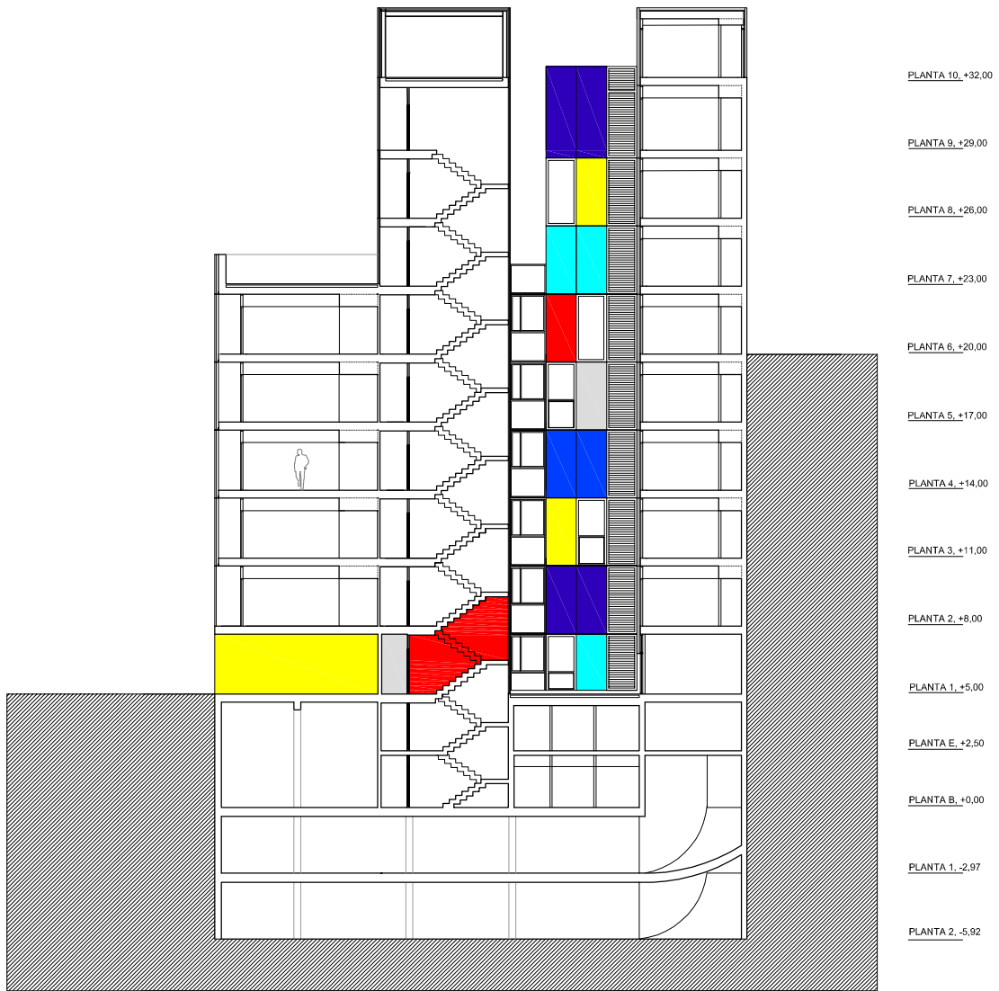
Seccion B-B'
