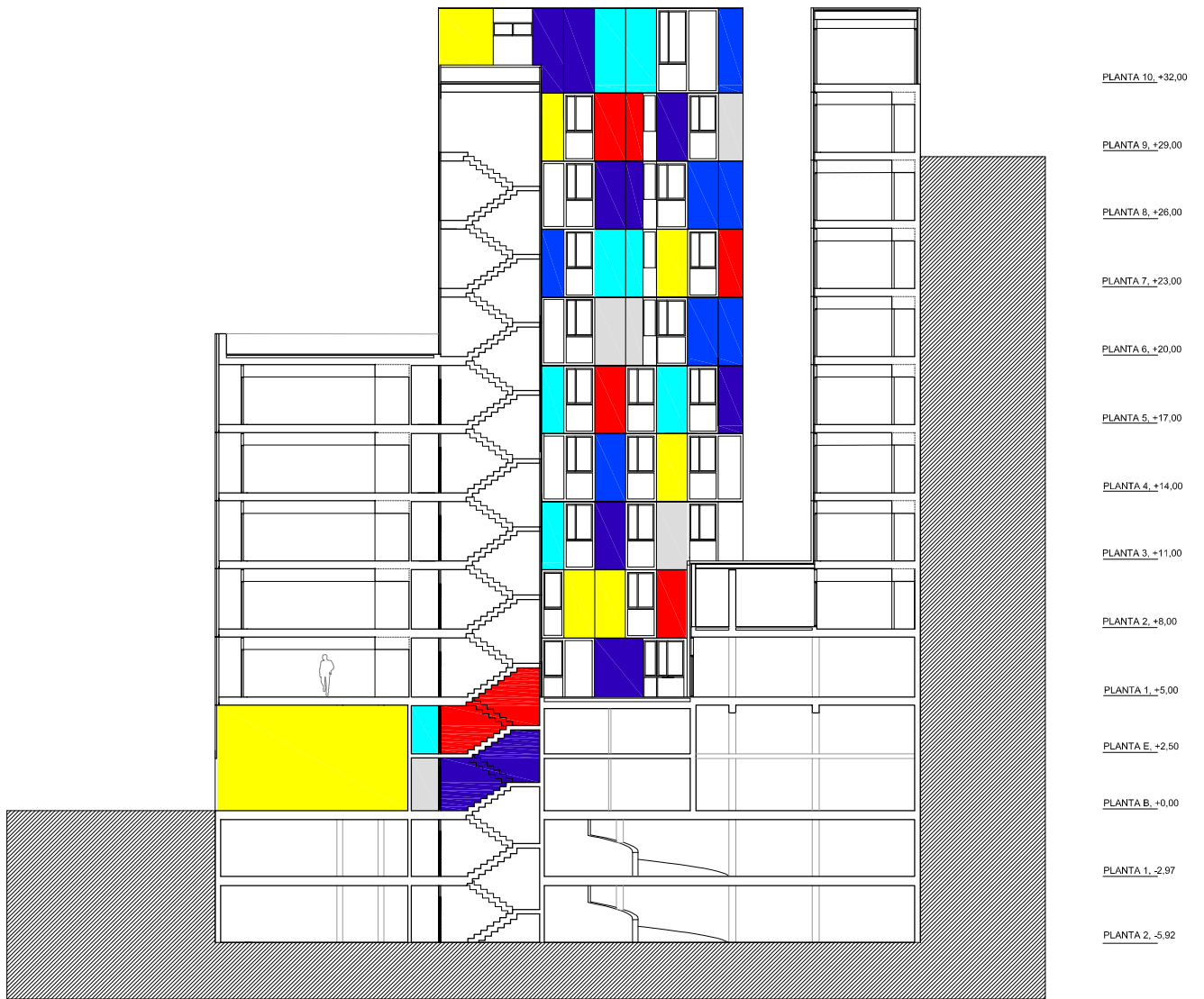
Seccion A-A'
