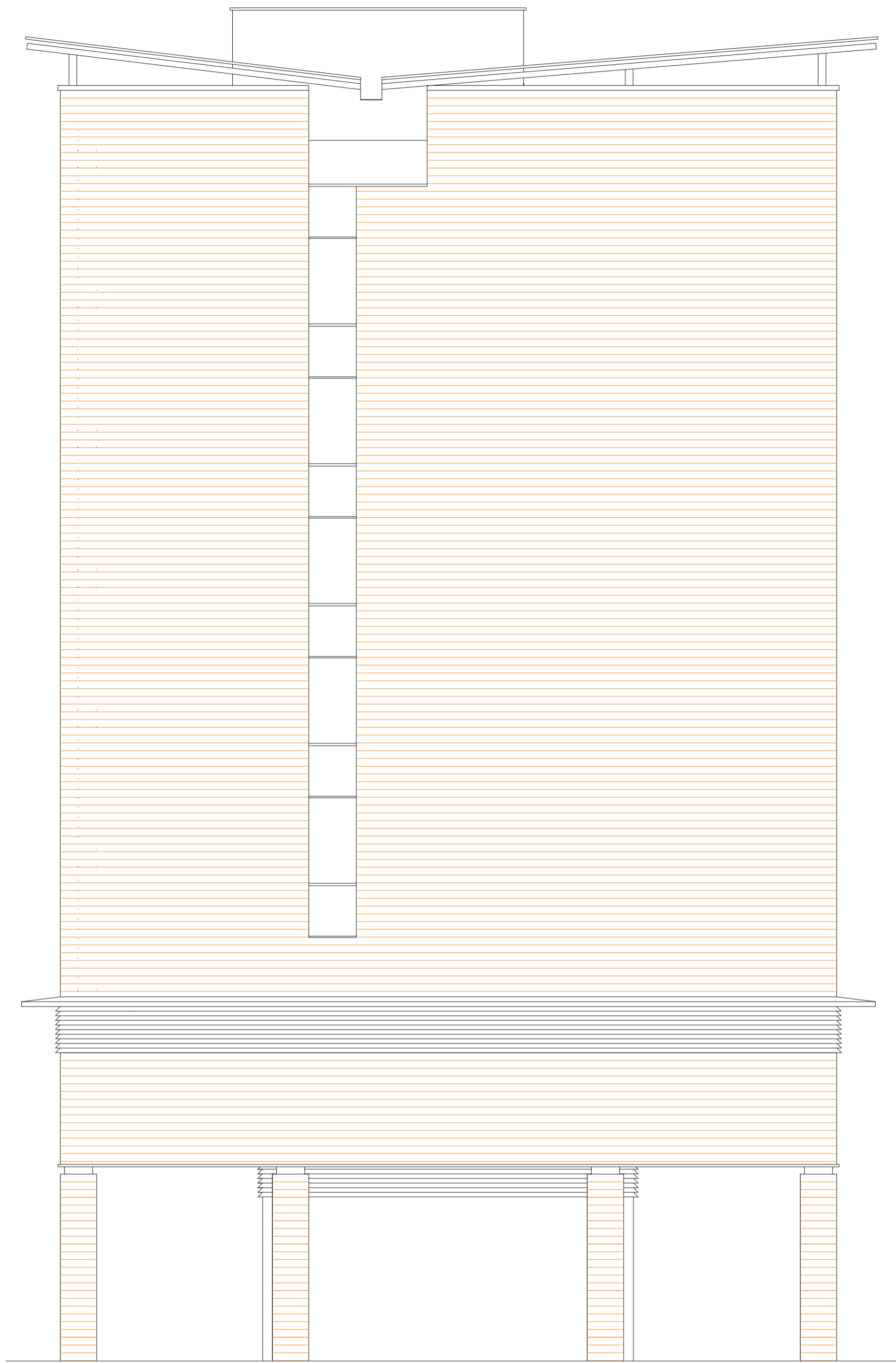
ALZADO SUR.
