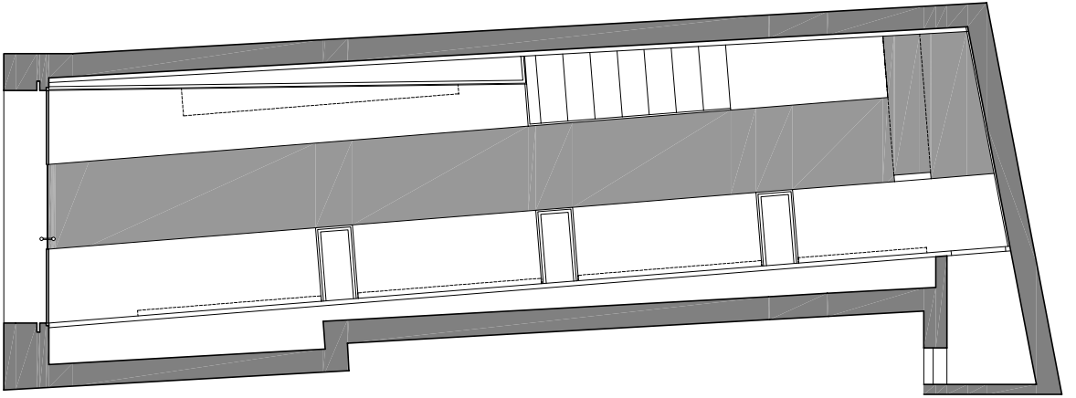
planta cota +0.80
