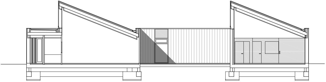
SECCIÓN A-A'
