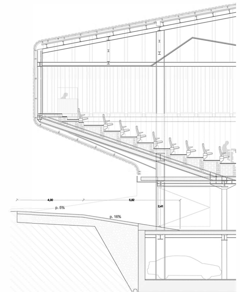
Detalle auditorio
