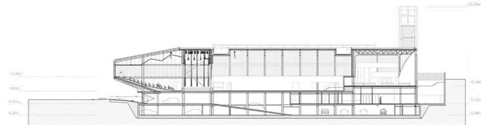
Sección B-B'
