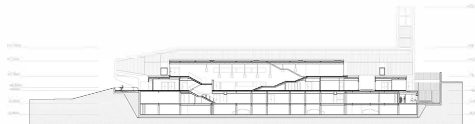
Sección C-C'
