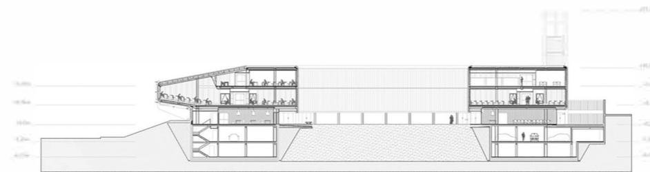
Sección A-A'
