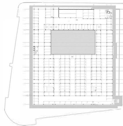
Planta Sótano
