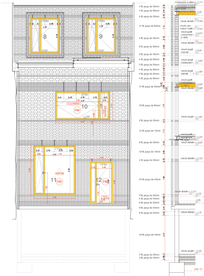
SECCIÓN C-C/ SECTION C-C
