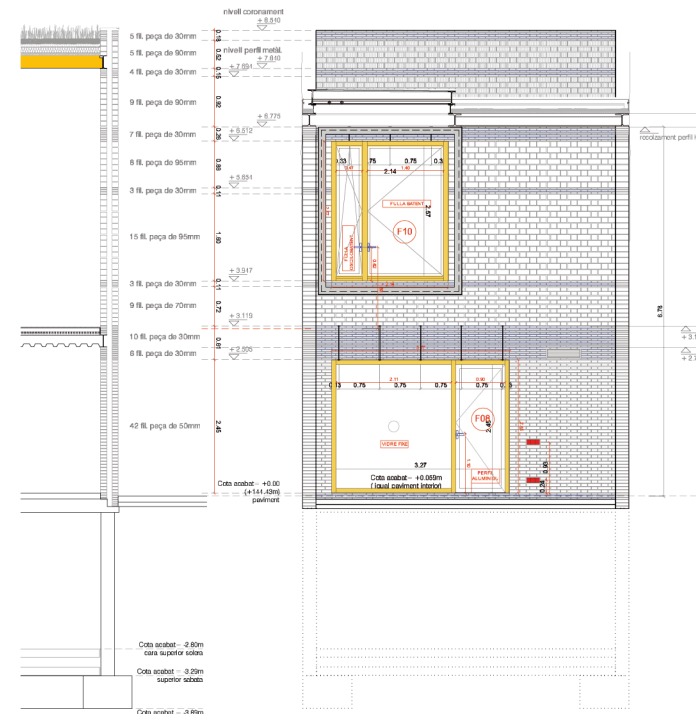
SECCIÓN F-F/ SECTION C-C
