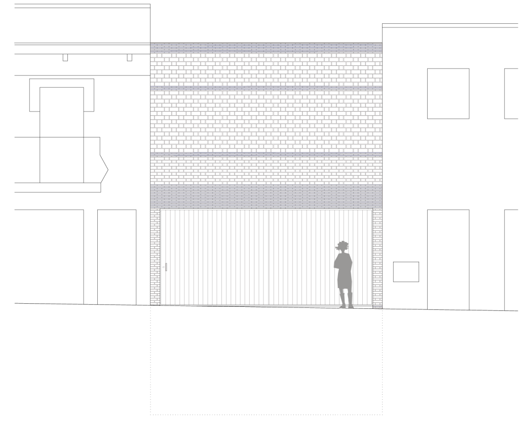
FACHADA DE LA CALLE MIQUEL RICOMÀ/ ELEVATION FROM MIQUEL RICOMÀ STREET
