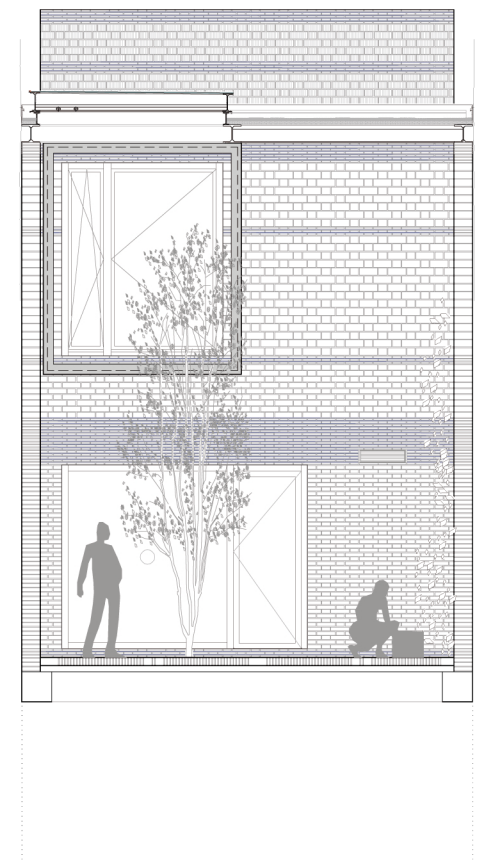
SECCIÓN F-F/ SECTION C-C'
