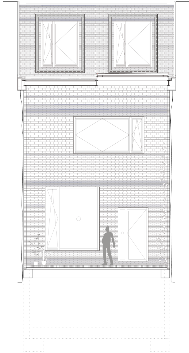
SECCIÓN C-C/ SECTION C-C'
