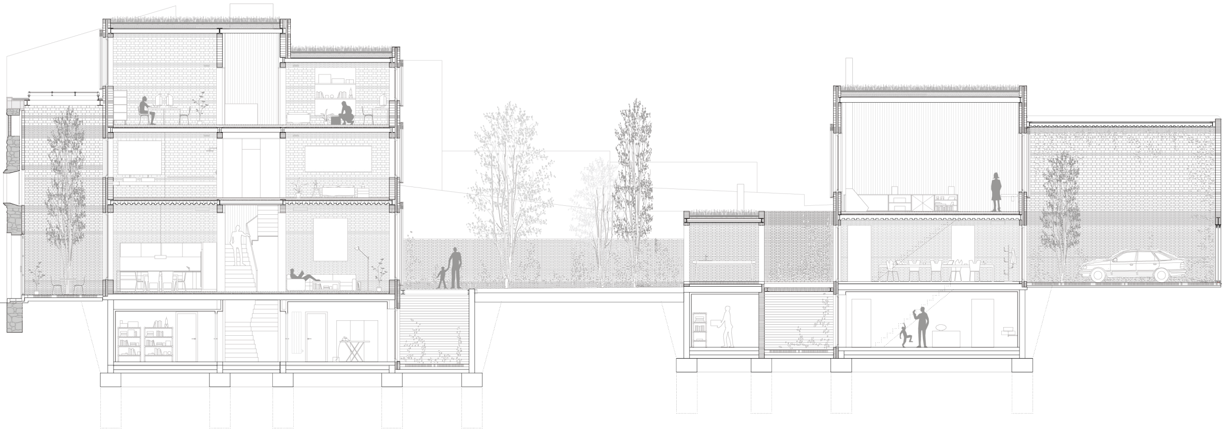
SECCIÓN A-A/ SECTION A-A'
