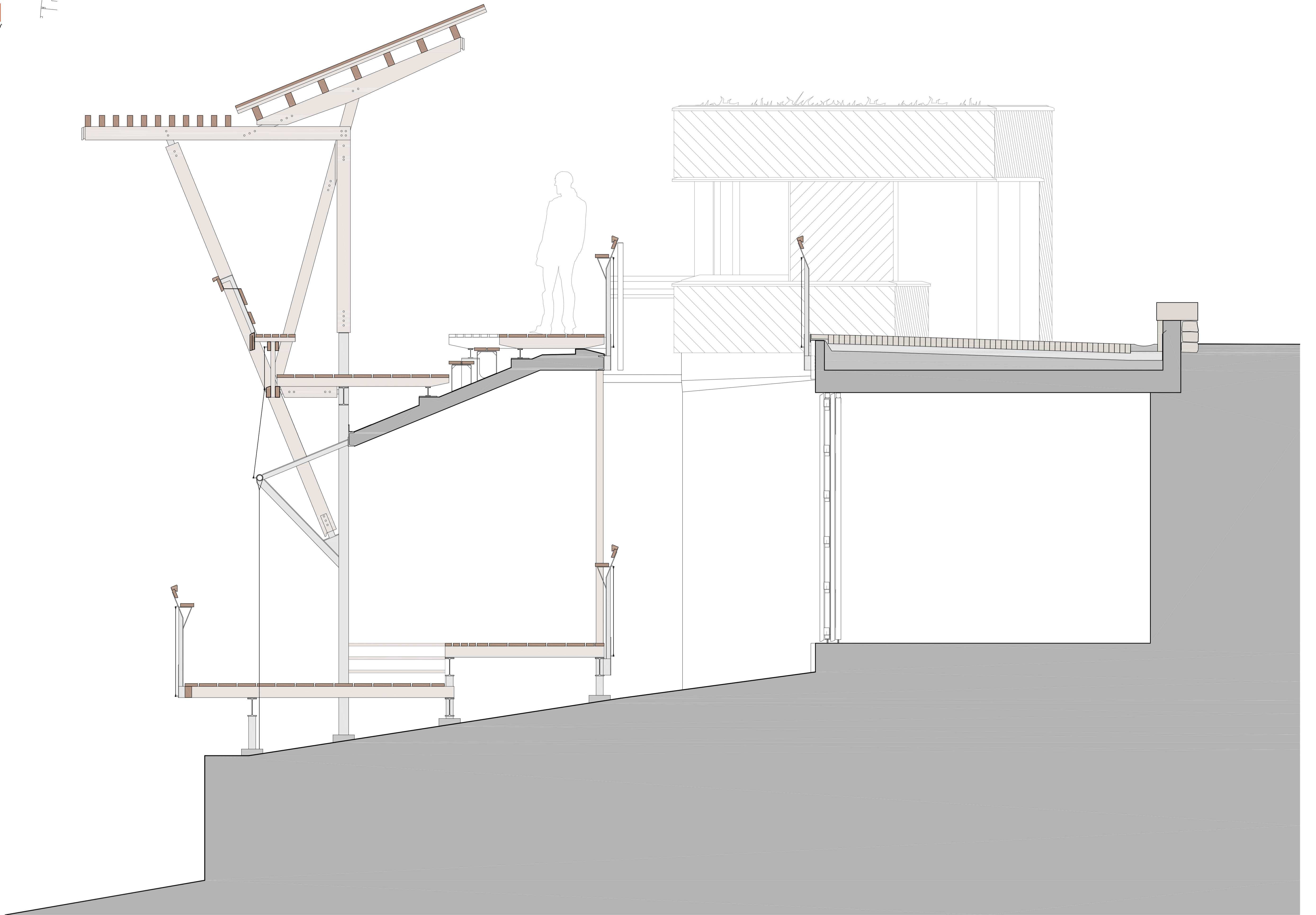
SECCIÓN DD' 0 0,5 1
