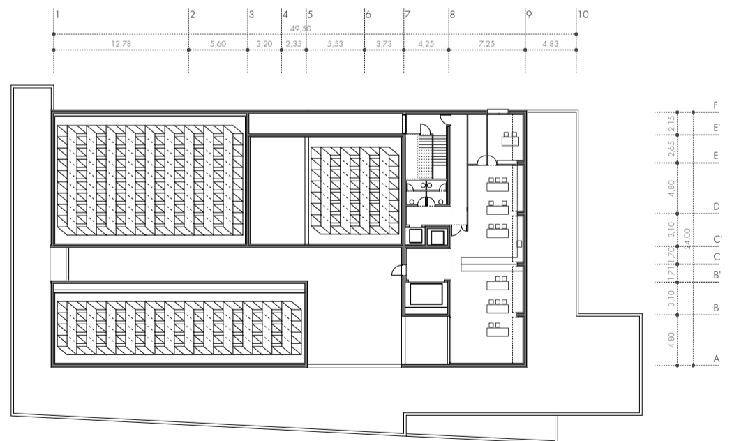
PLANTA CUARTA. LABORATORIO DE RESTAURACIÓN cota +15,30 LEVEL 4. RESTORATION WORKSHOP
