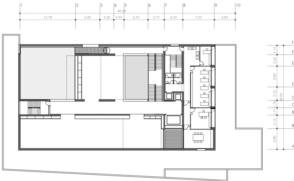
PLANTA SEGUNDA. SALAS. DIRECCIÓN cota +7,82 LEVEL 2. EXHIBITION ROOMS. OFFICES
