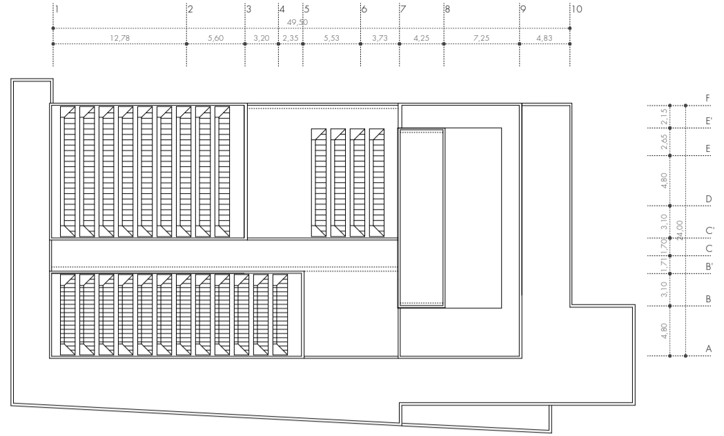
PLANTA DE CUBIERTAS ROOF PLAN
