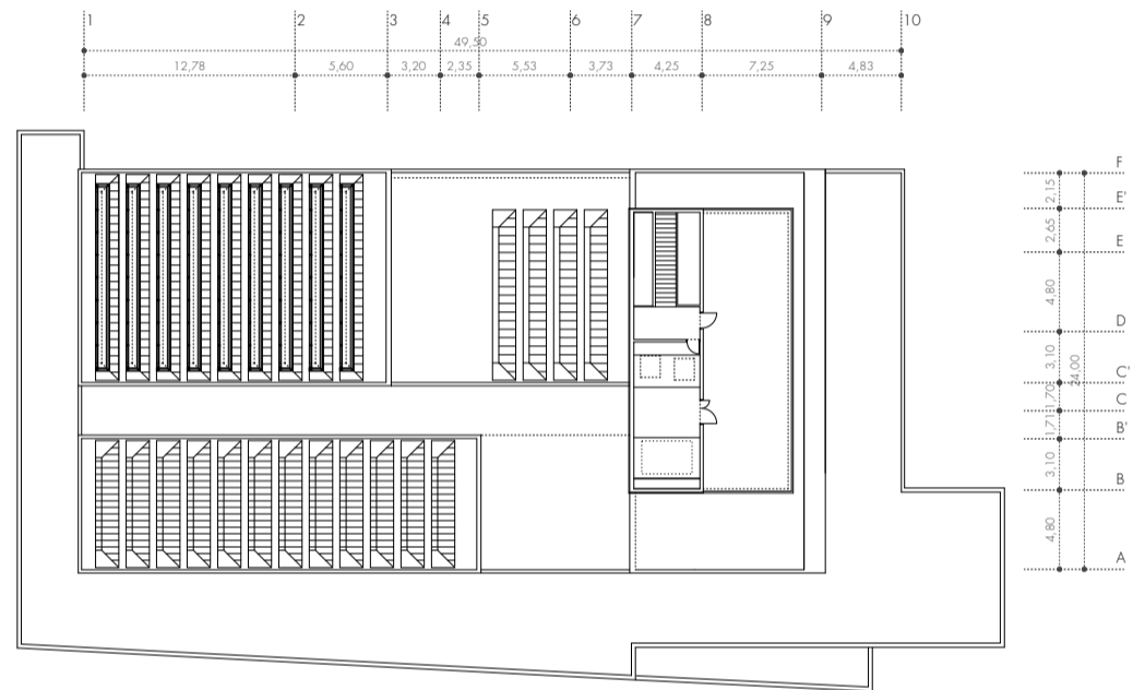
PLANTA QUINTA. LUCERNARIOS cota +19,04 LEVEL 5. SKYLIGHTS
