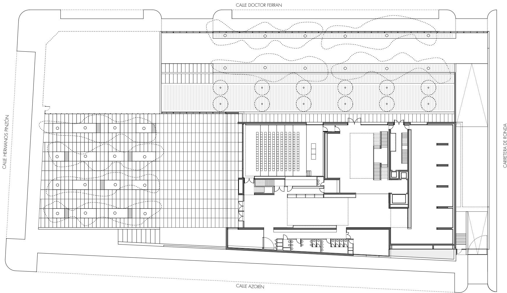
PLANTA BAJA. ACCESO AL MUSEO cota ±0,00 GROUND FLOOR PLAN. ENTRANCE
