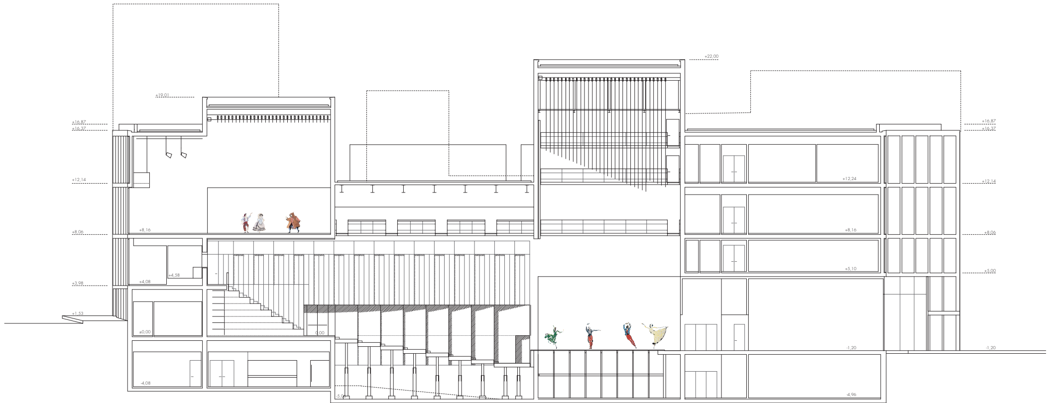
SECCIÓN LONGITUDINAL POR SALA
